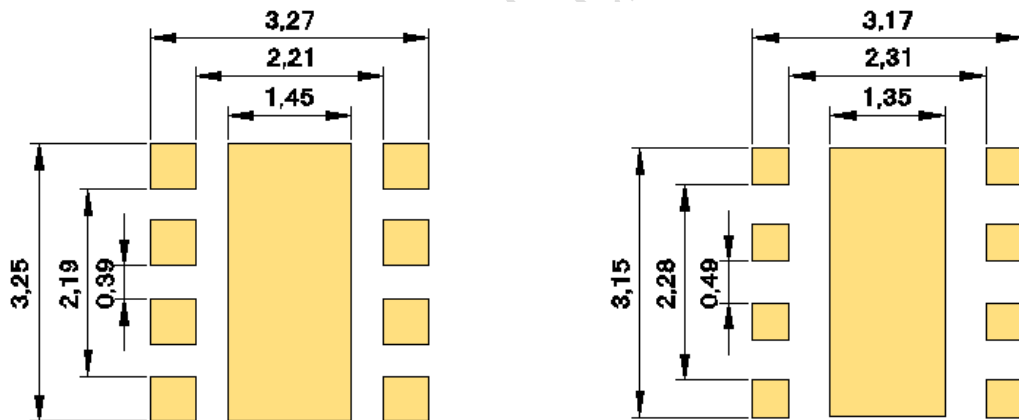
建议焊盘图
