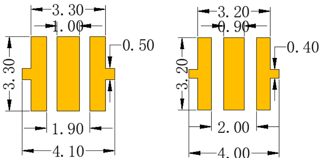
建议 PCB 焊盘
